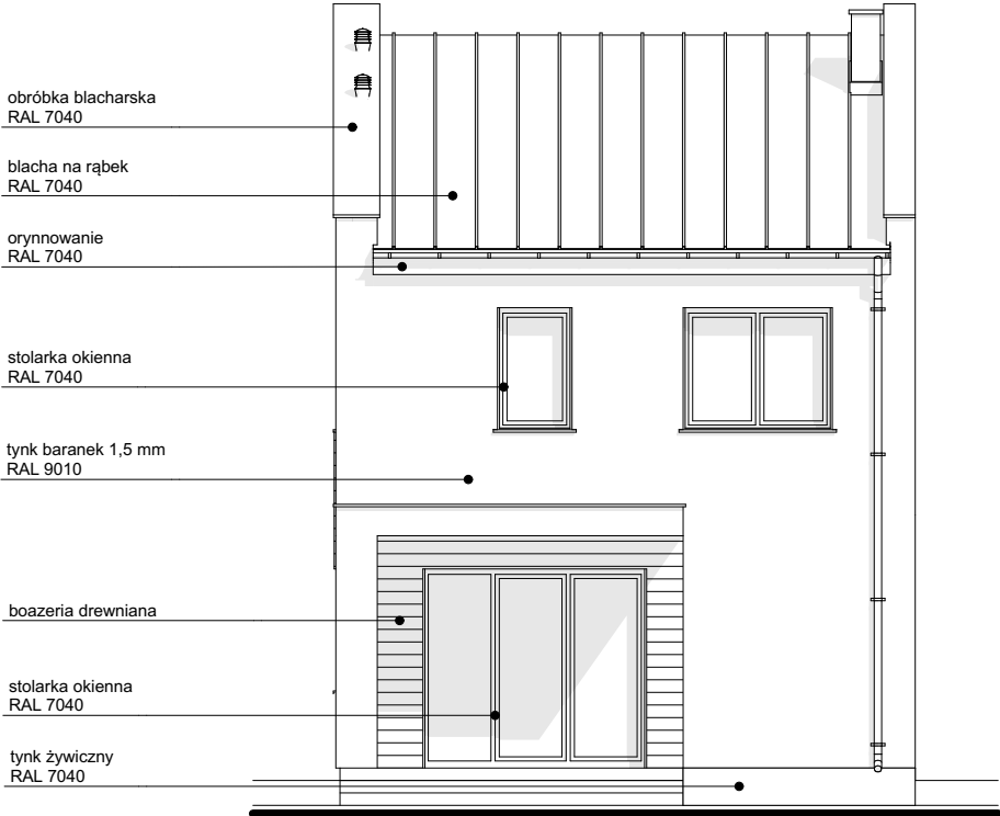
ELEWACJA POŁUDNIOWA
