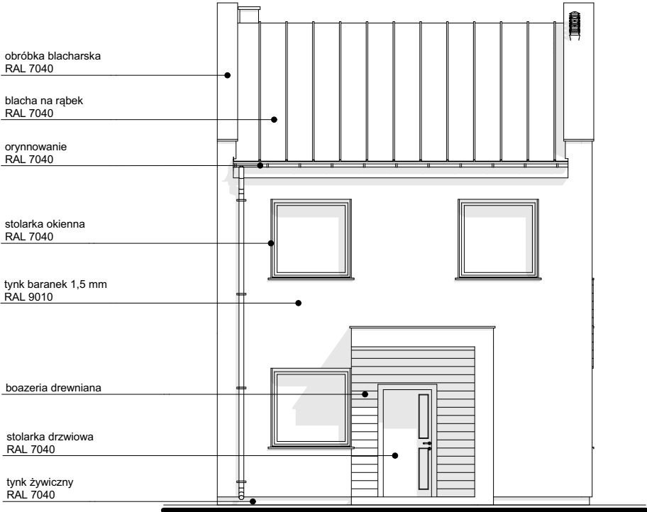
ELEWACJA PÓŁNOCNA
